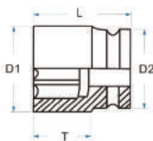
KPT-IS411 10PCS 1/2" Impact Sockets Set
